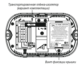
Рисунок 4. Светильника CA-7008Б. Вид сзади
